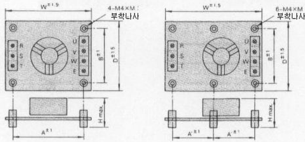
외형도 1
