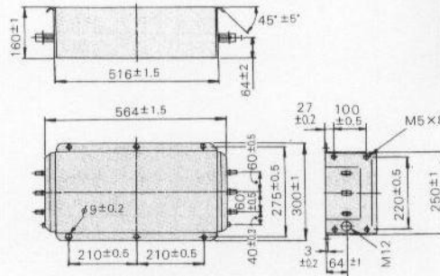
외형도 4
