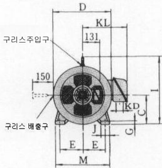
외형도 3
