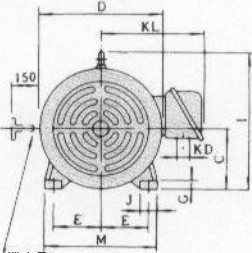
외형도 3
