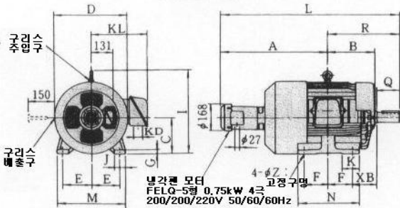
외형도 5
