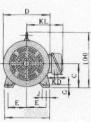
외형도 2
