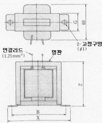
외형도 1
