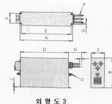
외형도 3
