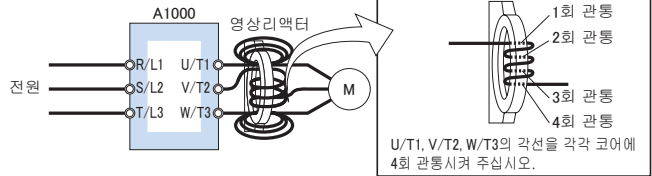
접속도 a
