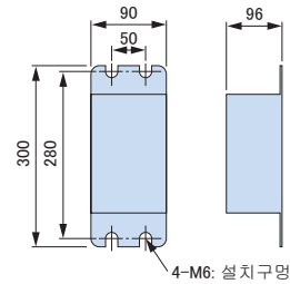
외형 크기 mm
