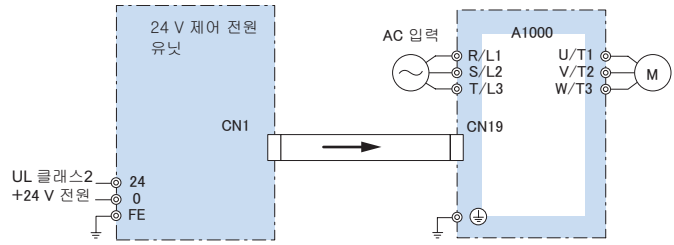
접속도
