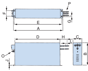
외형도 1
