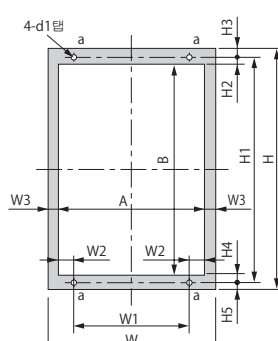
패널 가공도 2
