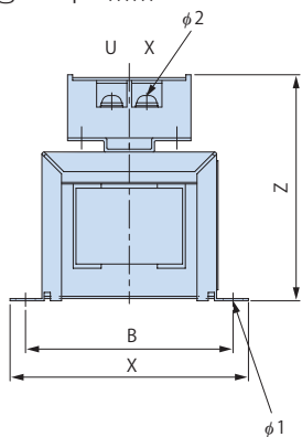
외형도 1
