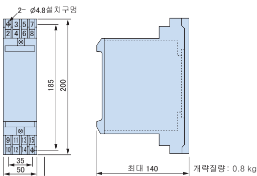
VS 시스템 모듈의 외형 크기 mm
