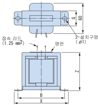
외형도 1
