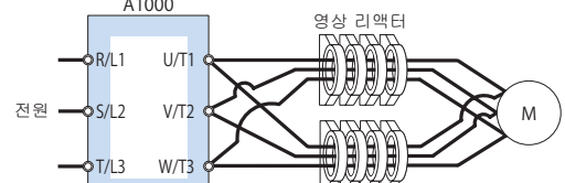
접속도 a
