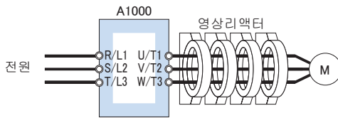
접속도 b
