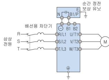
접속도
