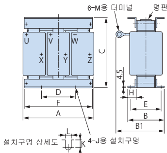
외형 크기 mm
