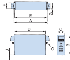
외형도 2
