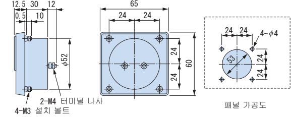
외형 크기 mm
